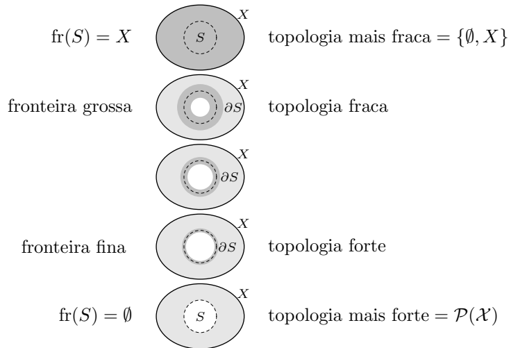
Figura 2.15: A influência da força da topologia na espessura da fronteira.
