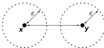
Figura 1.3: Dois pontos distintos x e y podem ser “separados” por bolas disjuntas.
