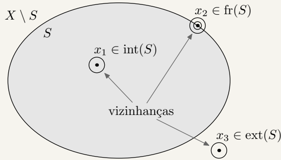
Figura 2.14: Interior, Exterior e Fronteira
