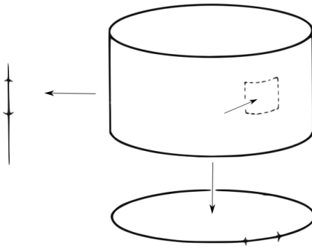
Figura 4.3: O cilindro é o produto de S^1 \times [0, 1]
