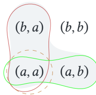
Figura 4.2: Topologia produto de dois espaços de Sierpiński.
