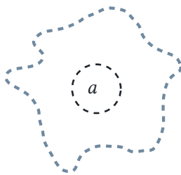
Figura 1.4: Em torno de cada ponto de um aberto cabe uma bola ainda contida nele.
