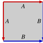
Figura 4.9: Um esquema de identificação que produz a esfera.
