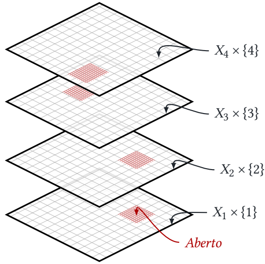
Figura 4.11: Soma de Espaços Topológicos
