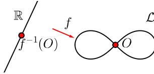
Figura 3.2: A lemniscata antecipa um argumento local que será formalizado por conexidade.
