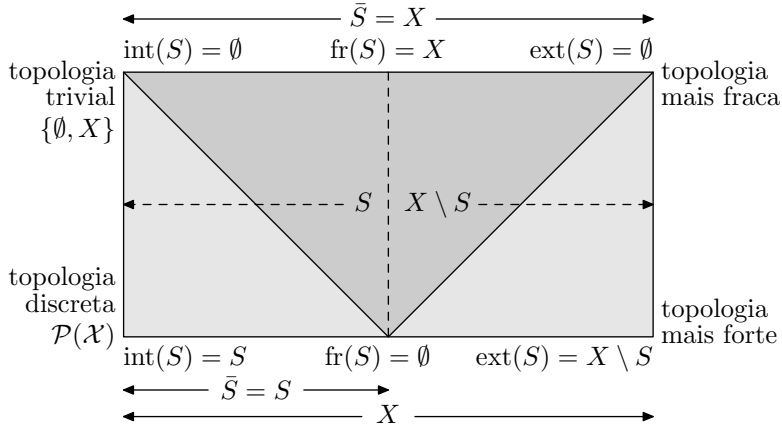
Figura 2.16: Interior, limite e exterior de conjuntos incluindo as topologias extremas discreta e trivial.
